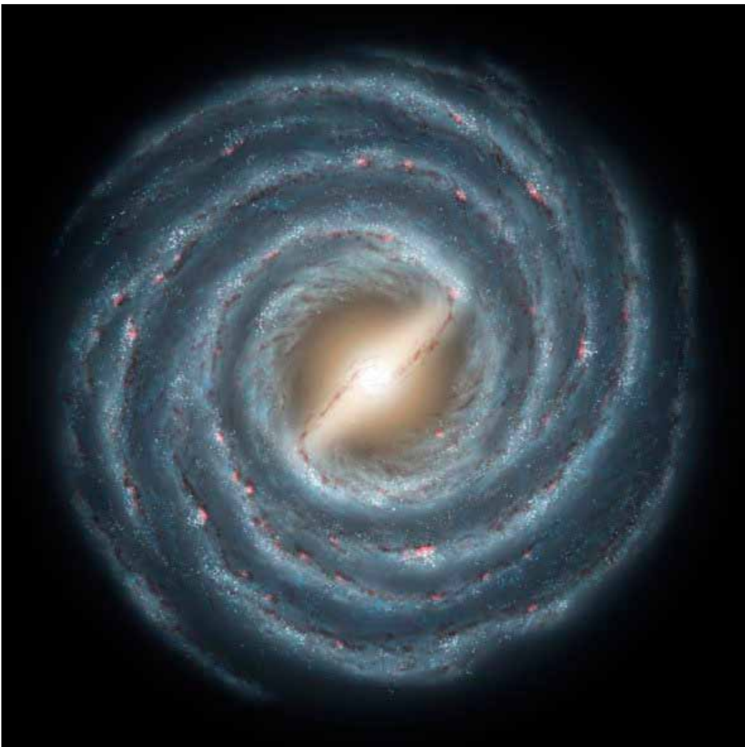
Stjärnorna i Vintergatan är fördelade i en tunn diskusskiva som har en spiralliknande form. I mitten finns en upphöjning, en bula, i form av en stav. Vintergatan kallas därför för en stavspiralgalax. Bilden visar hur Vintergatan skulle kunna se ut på stort avstånd högt ovanför den diskusformiga skivan. FOTO: NASA
